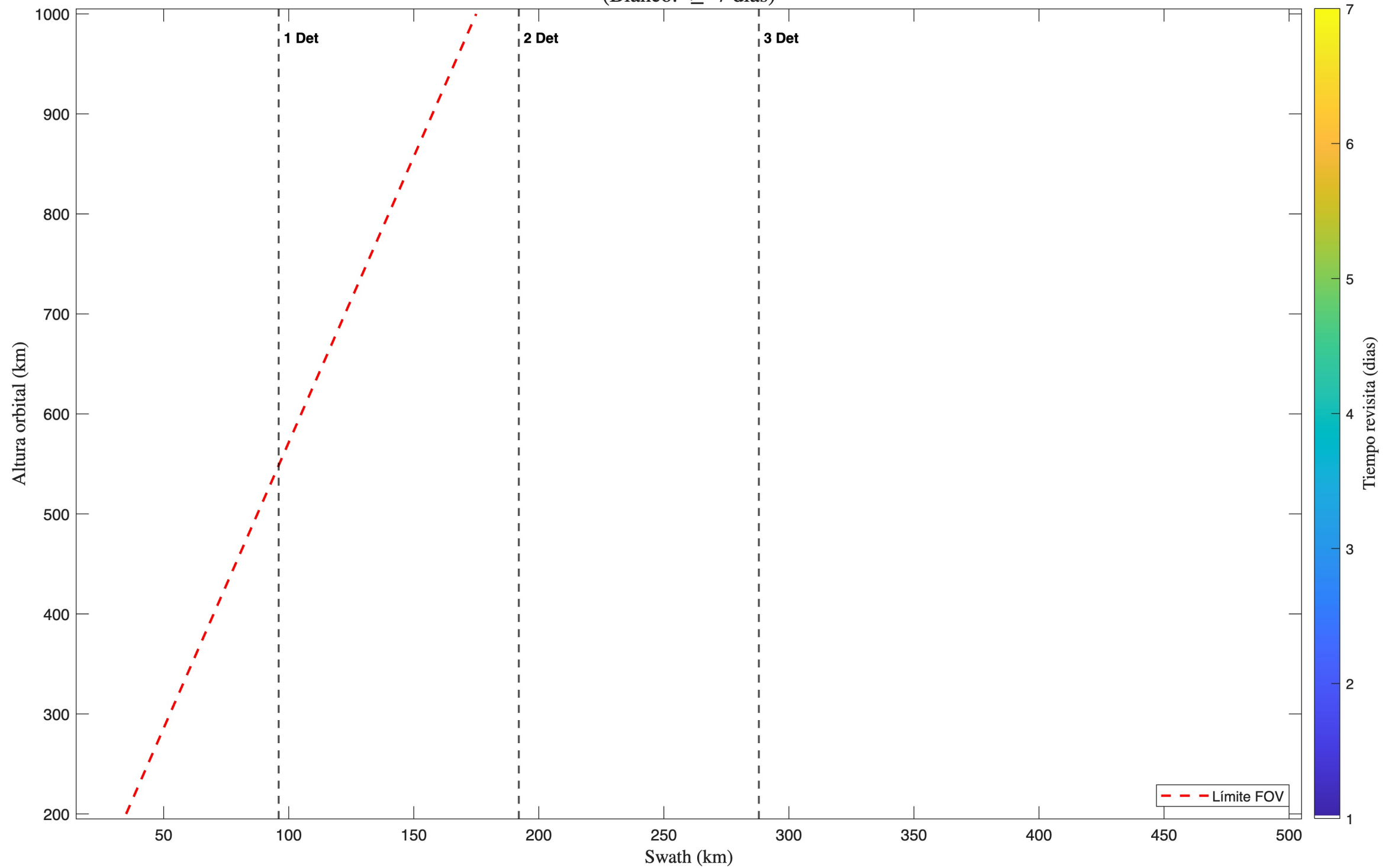
Tiempo Revisita - 2 Satellite(s); 1 Telescopio(s): Refractivo; Detector 1 (Blanco: \geq 7 días)
